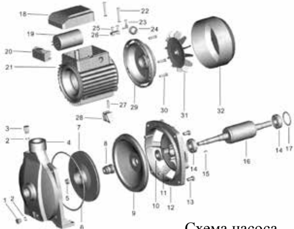
Схема насоса
